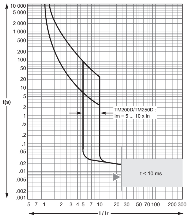
TM200D / TM250D
