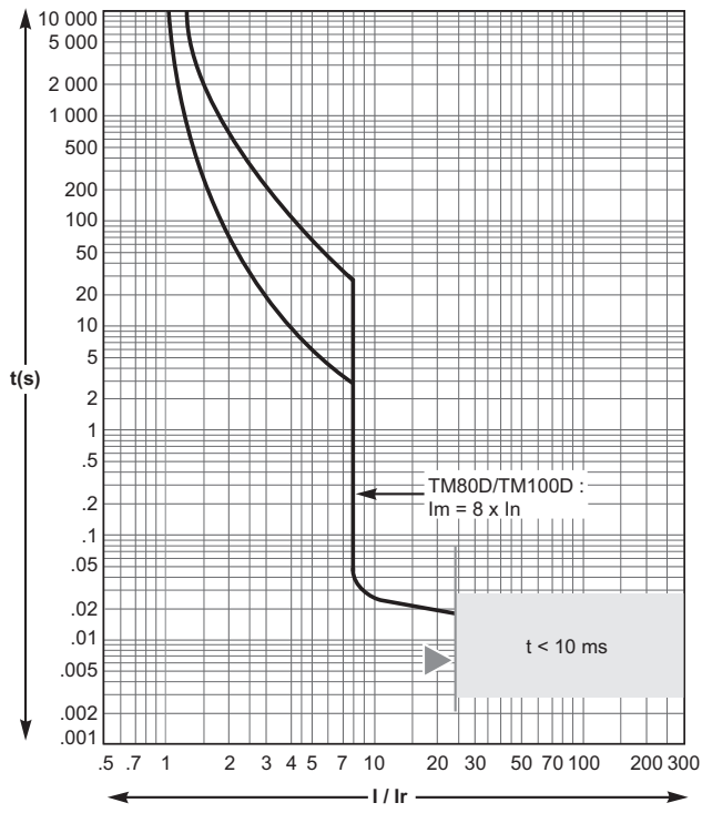
TM80D / TM100D
