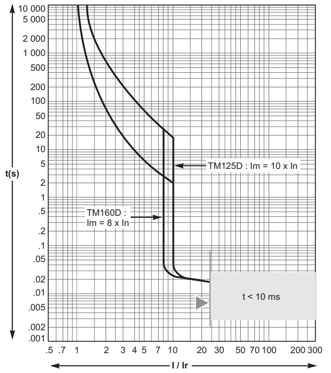
TM125D / TM160D
